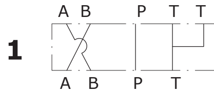
Hidraulikus ábra
